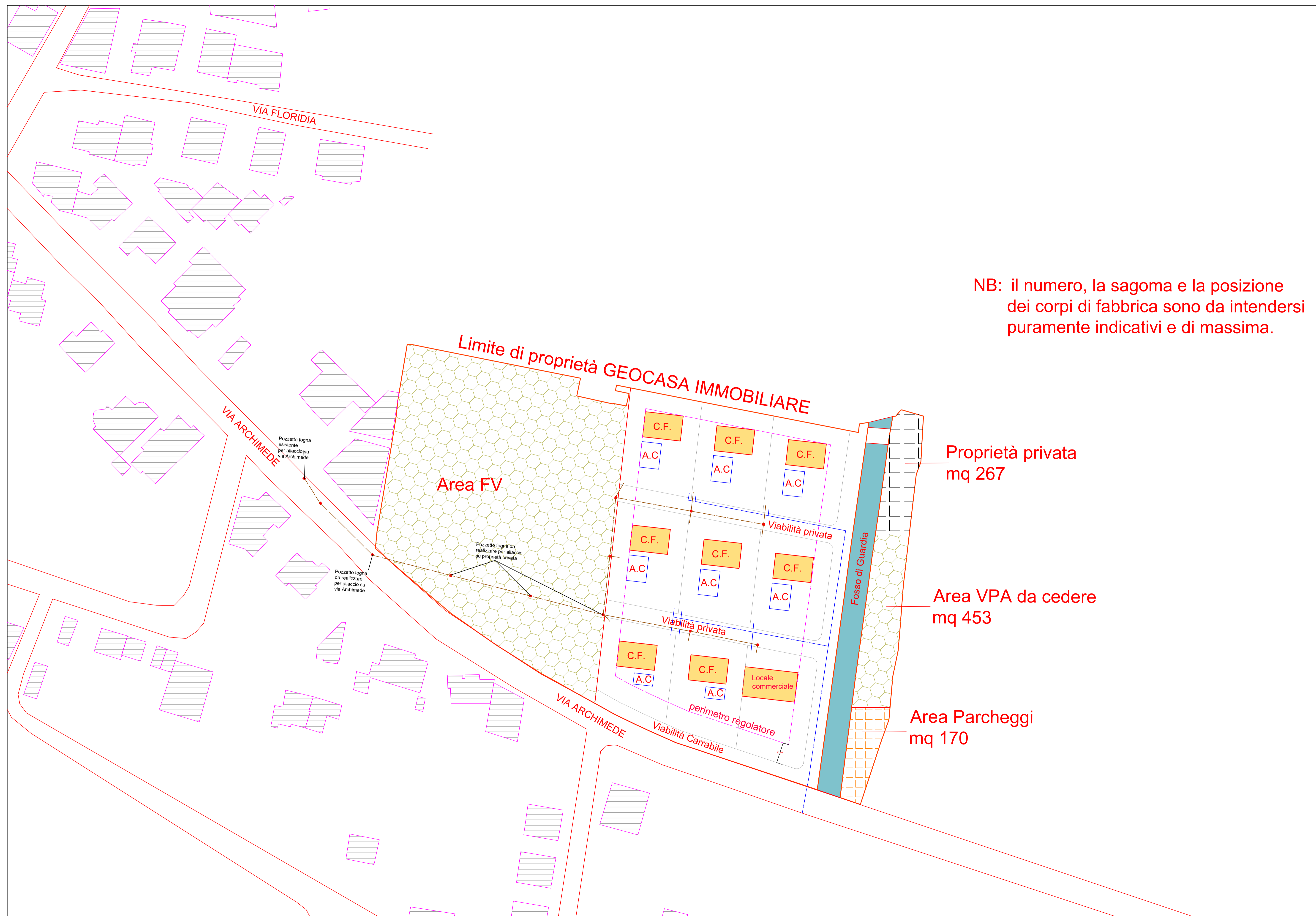
Planimetria Allaccio Fognario e Idrico scala 1:500
