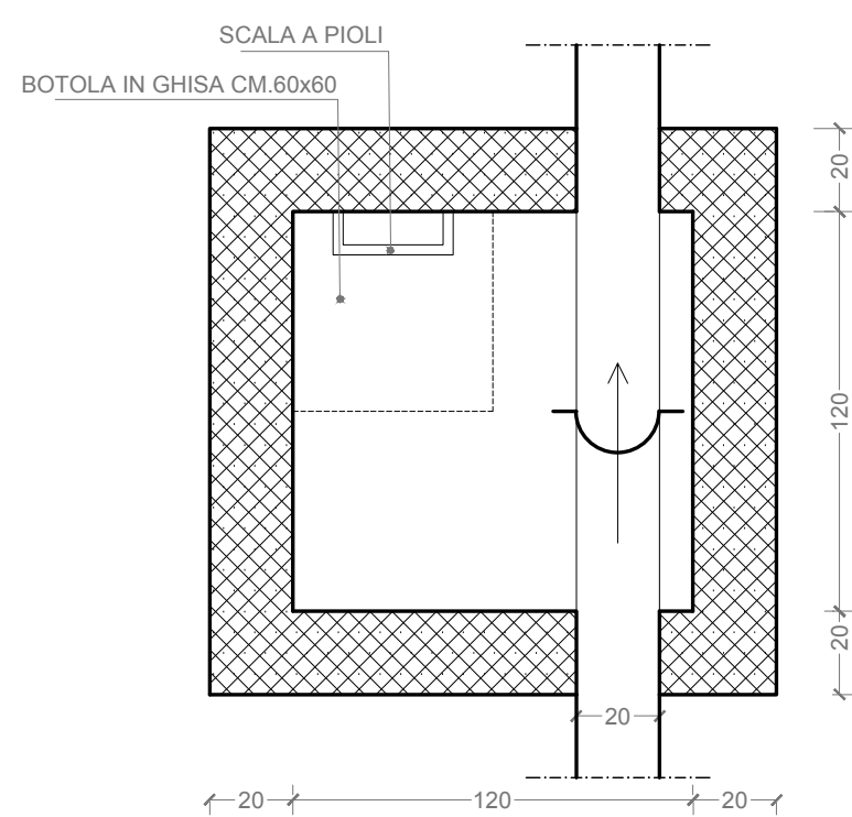
POZZETTO IN LINEA ACQUE NERE PIANTA 1:25
