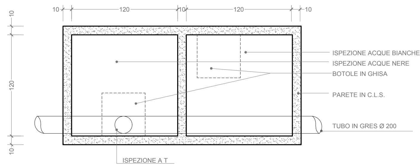
PIANTA POZZETTI D'ISPEZIONE 1:25
