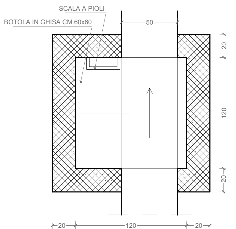
POZZETTO IN LINEA ACQUE BIANCHE PIANTA 1:25
