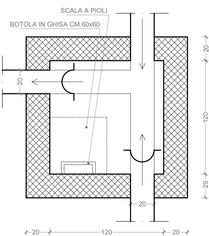
POZZETTO INCROCIO ACQUE NERE PIANTA 1:25
