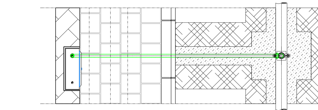
Allacci alla rete idrica da acquedotto comunale 1:20
