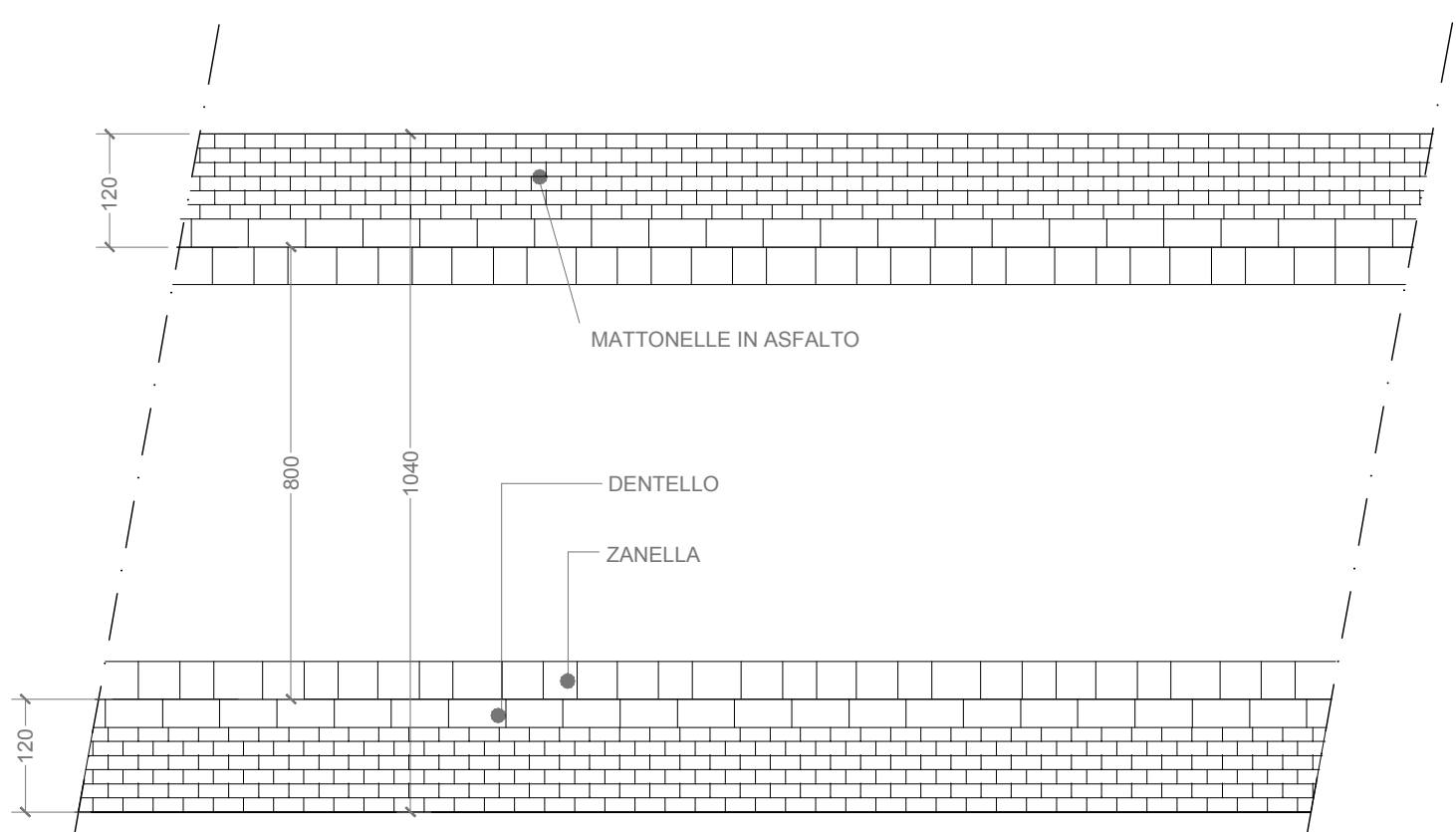
PARTICOLARE CARREGGIATA - PIANTA 1:100
