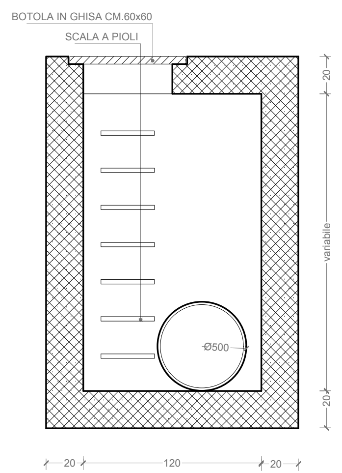
POZZETTO IN LINEA ACQUE BIANCHE SEZIONE 1:25
