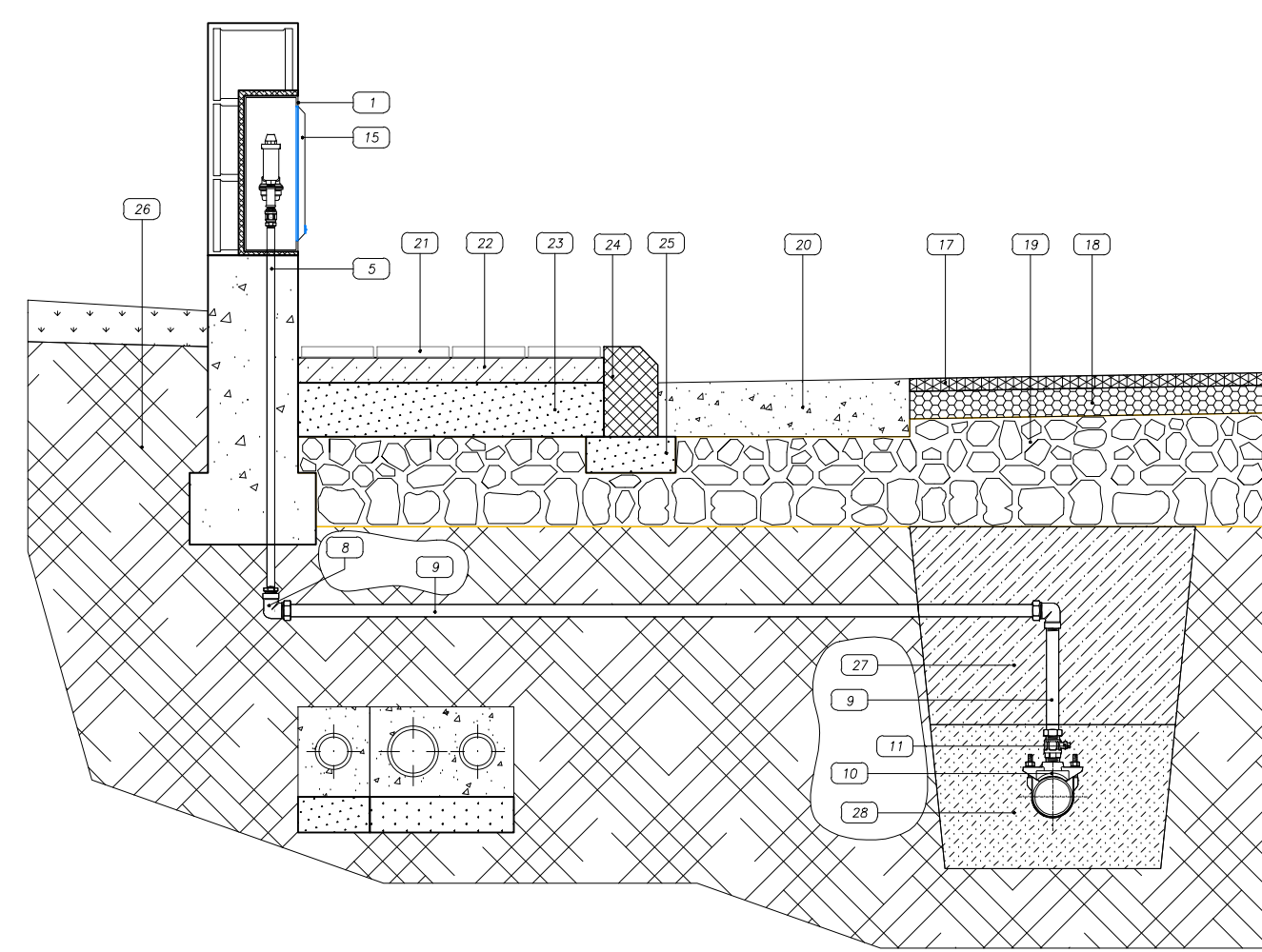
Derivazioni allacci privati con collare di presa 1:20
