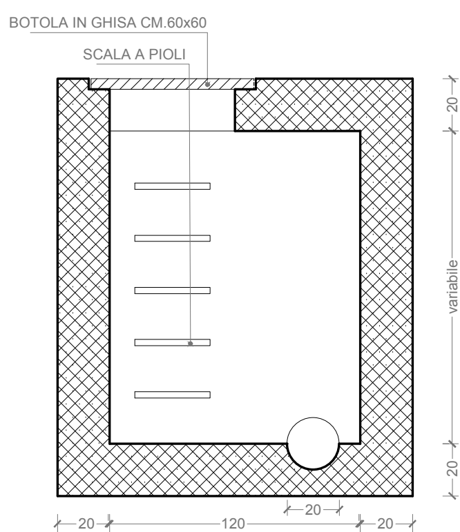
POZZETTO IN LINEA ACQUE NERE SEZIONE 1:25
