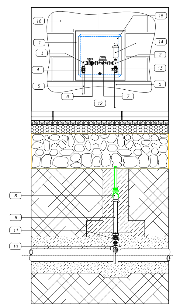
Gruppo contatore - utenza singola 1:20
