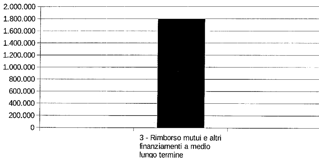
Diagramma 11: Indebitamento
